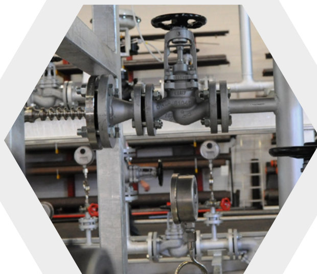
3. Industria chimica per la produzione di solventi. Particolare skid processo Fase 2 completo di supporto, valvole e strumentazione.
